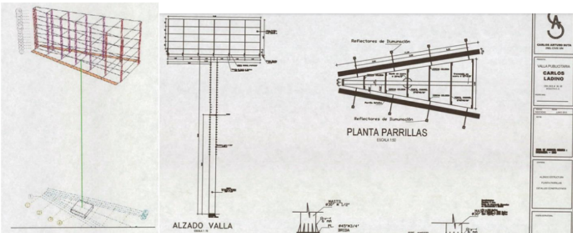
Imagen 1. Estructura calculada y diseñada. Tomado del radicado 2014ER136282.
